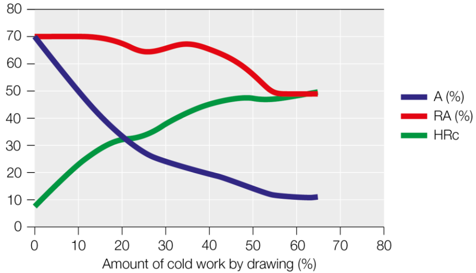
Figure 3 Allongement A (%) Striction RA (%) Dureté HRc Etat écroui à froid
