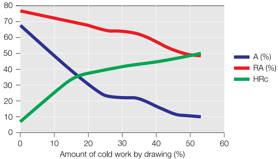
Figure 4 Allongement A (%) Striction RA (%) Dureté HRc Etat écroui à froid + vieillissement
