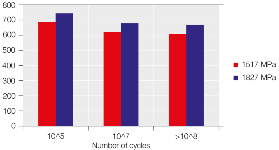
Figure 5 Fatigue en flexion rotative selon Moore Etat écroui à froid + vieillessement
