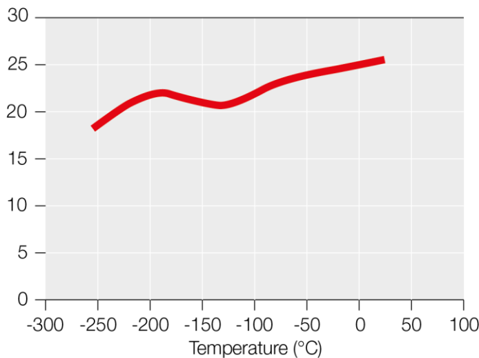
Figure 6 Résilience selon Charpy V-notch (J)
